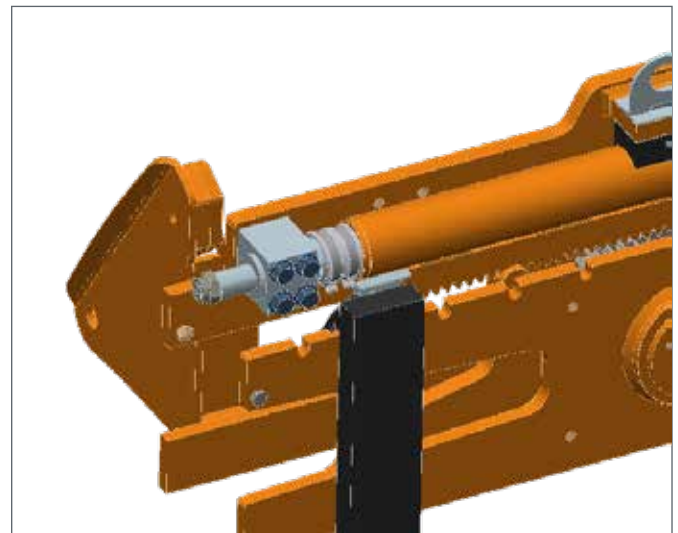
Anschlag Position 0°
